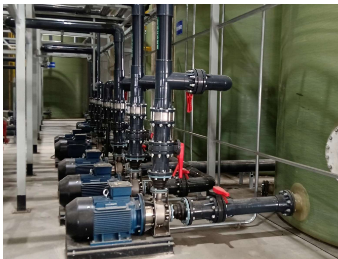
Xử lý nước môi trường
